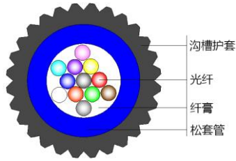
a. 中心管式
