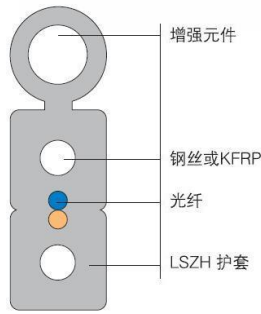
b. 自承架空型
