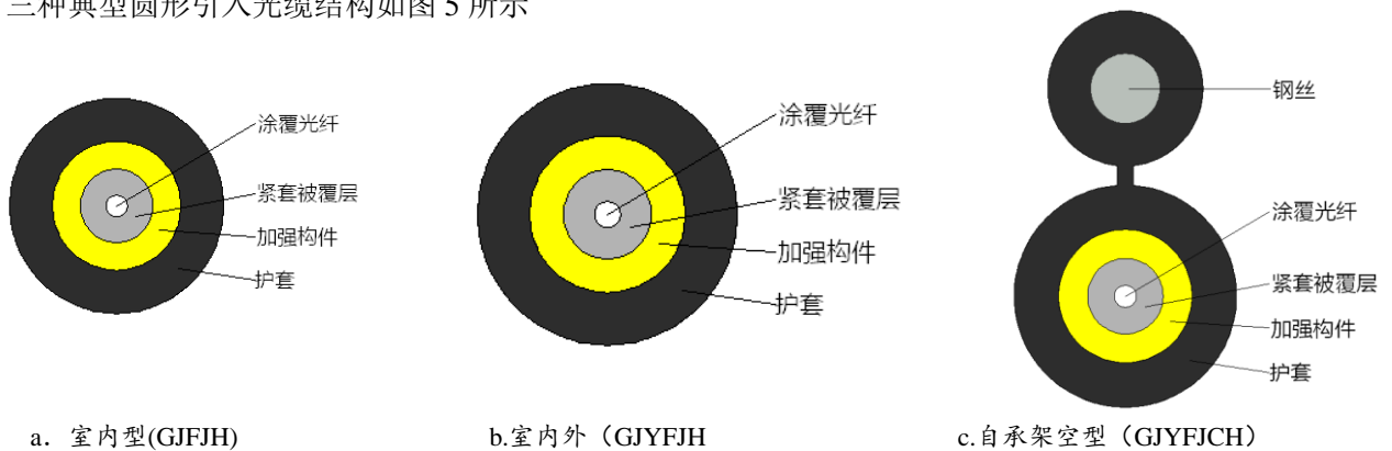
图 5 圆形引入光缆典型结构图
