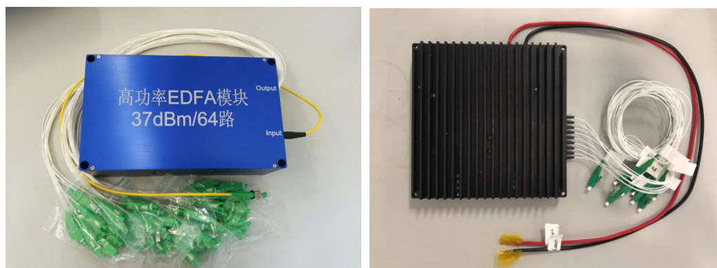
图 2 (a) 广电市场高功率 EDFA 模块 (b)广电市场高功率 EDFA Gain Block
