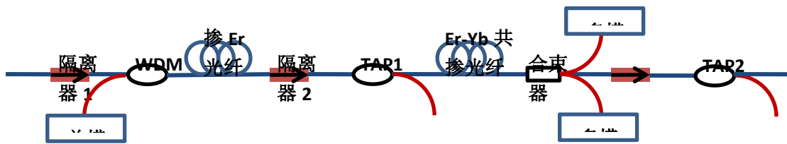
图 1 中高功率 EDFA 模块原理图
