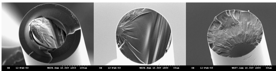
图 2 光纤在不同应力下的断裂端面图（应力从左到右变小）
