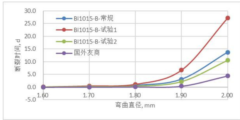
图 5 极小弯曲半径下，国内外弯曲不敏感光纤断裂时间对比
