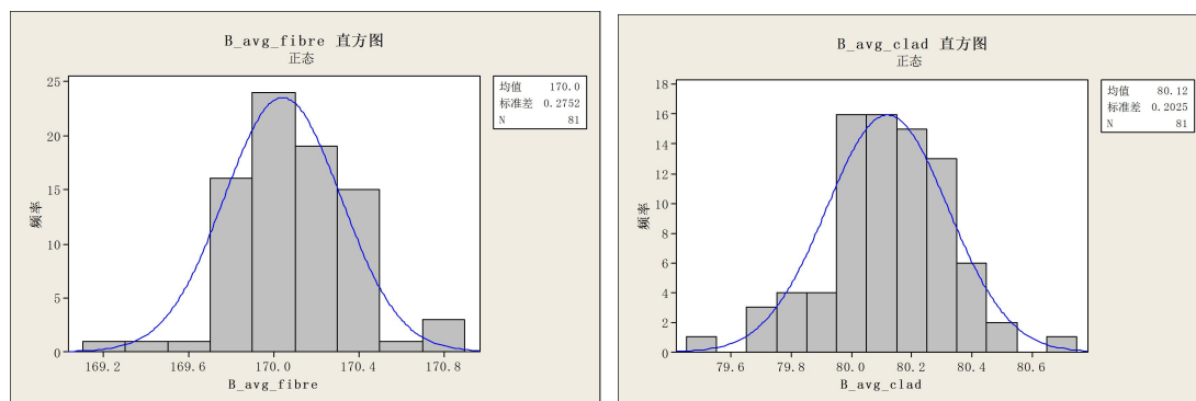
图 3 长飞公司 BI1015-B 系列光纤涂覆层和包层统计数据
