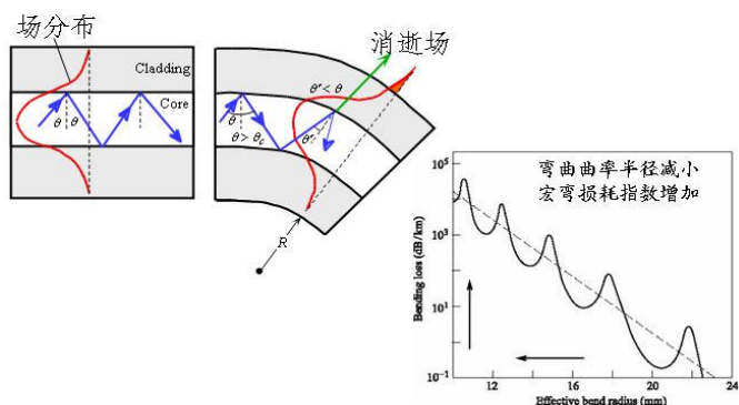
图 1 弯曲导致的光纤损耗原理图
