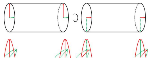
图1 旋转光纤保圆机理示意图
