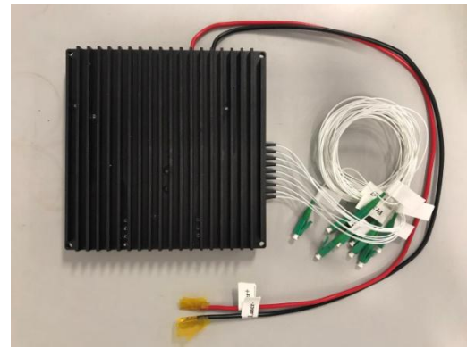
图 2 (a) 广电市场高功率 EDFA 模块 (b) 广电市场高功率 EDFA Gain Block
