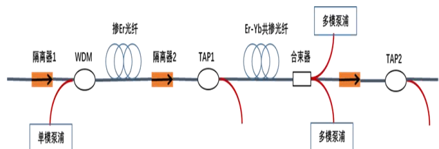
图 1 中高功率 EDFA 模块原理图
