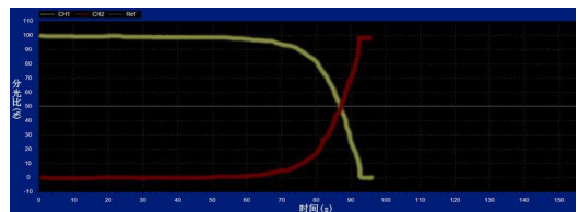
图 1 采用长飞细径 CS980 拉制 980/1550 WDM 980nm 和 1550nm 波长波形图 (图中黄线为 980nm 分光比，红线为 1550nm 分光比)
