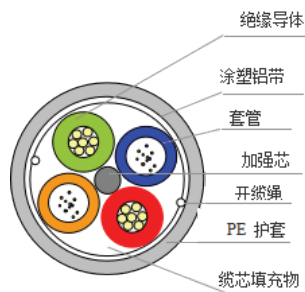
图1 GDTA—24 Xn+2*6.0
