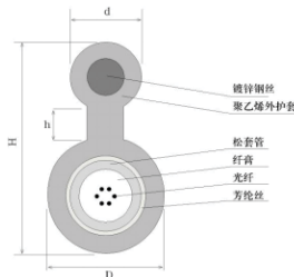
图1 GYAXTC8Y—2~12Xn
