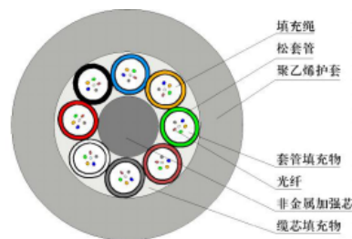
图1 GYFTY-48Xn
