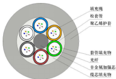
图1 GYFTY-36Xn
