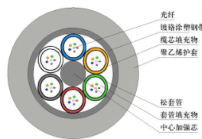
图2 GYTS-36Xn
