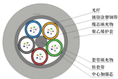
图1 GYTS-30Xn
