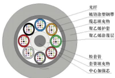
图3 GYTS-96Xn
