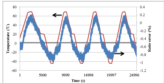
图 2 客户验证的长飞旋转光纤的比差 VS 温度线性度
