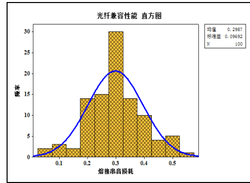
图 2 光纤兼容性
