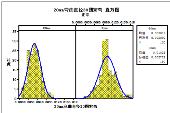
图 4 宏弯性能
