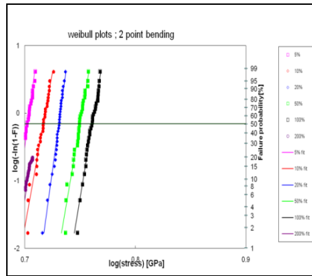
图 5 机械强度
